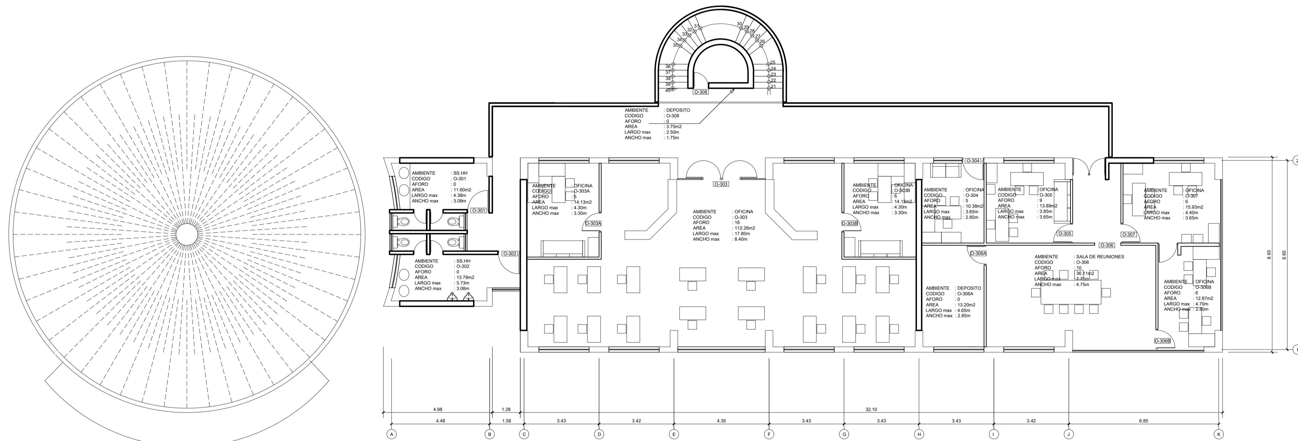
TERCERA PLANTA AREA TECHADA = 431.83m 2 AFORO = 64 ESCALA 1:100
